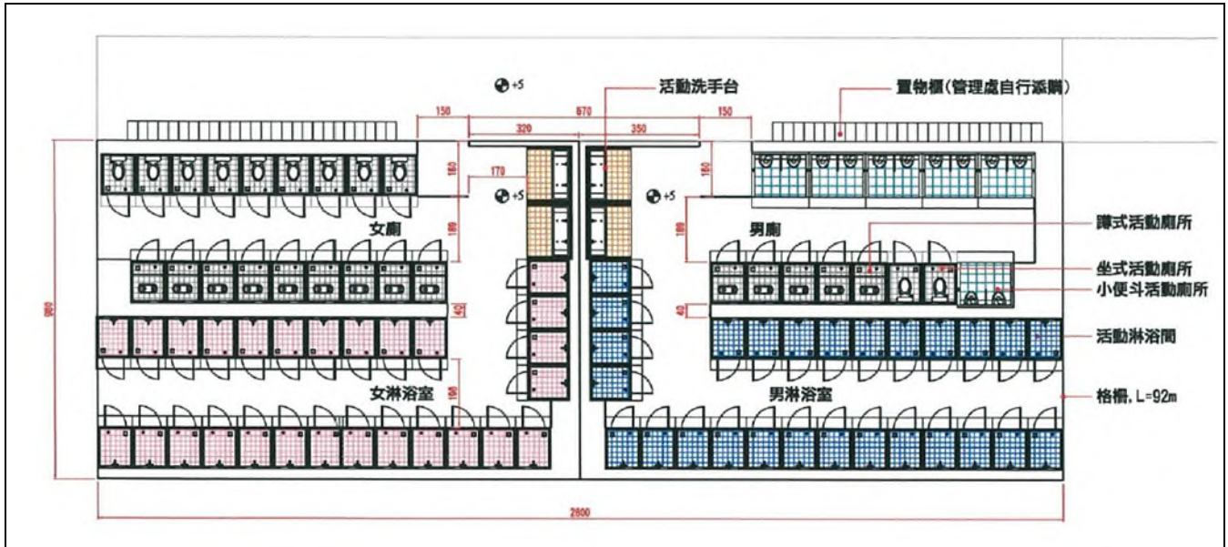
圖 3：土壟灣遊客服務區-廁所平面圖
