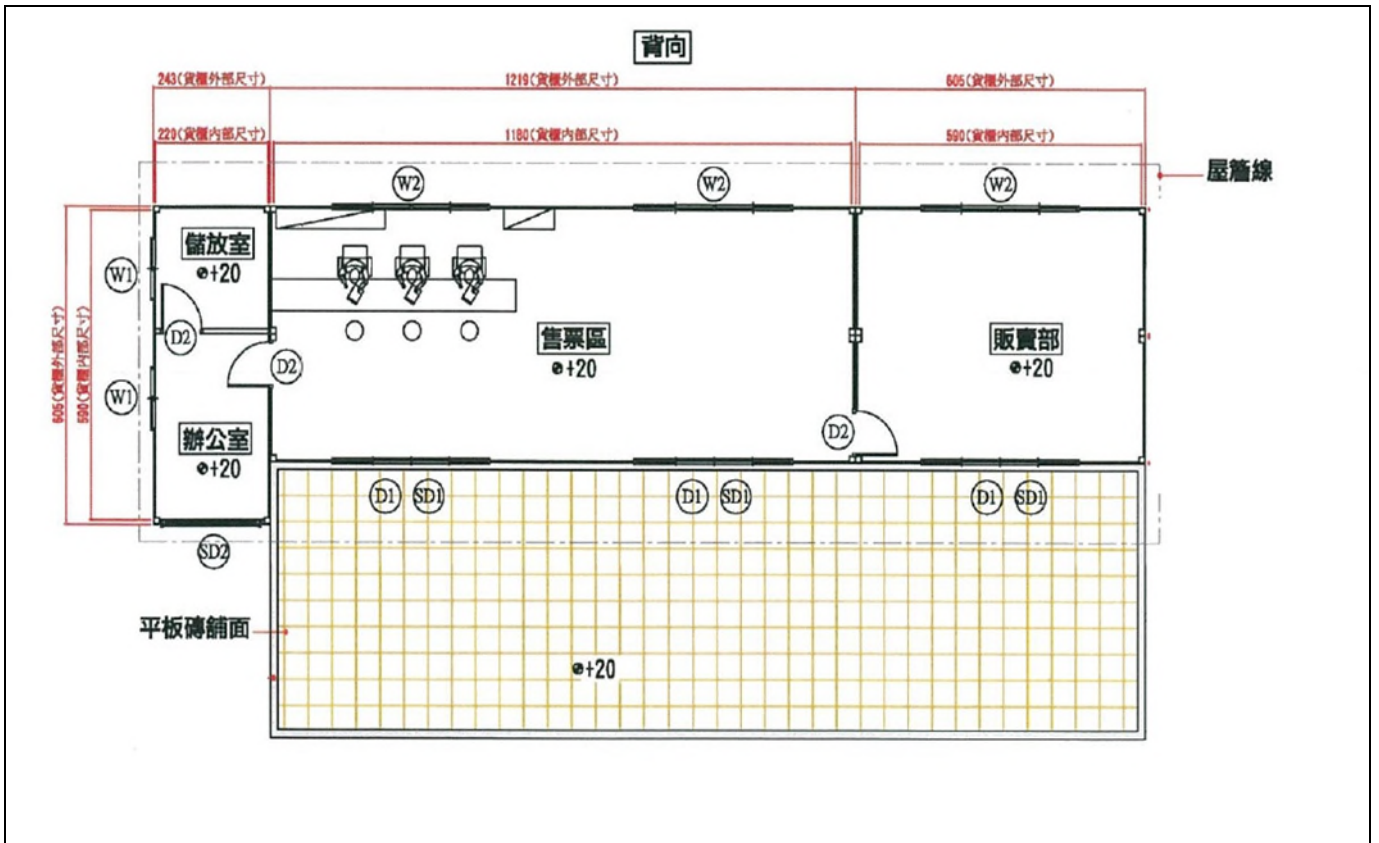
圖 2：土壟灣遊客服務區-辦公室平面圖
