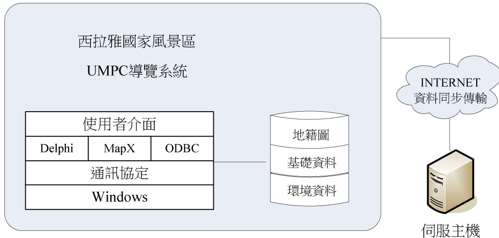
圖 3-5 UMPC 導覽系統整體之資訊架構圖
