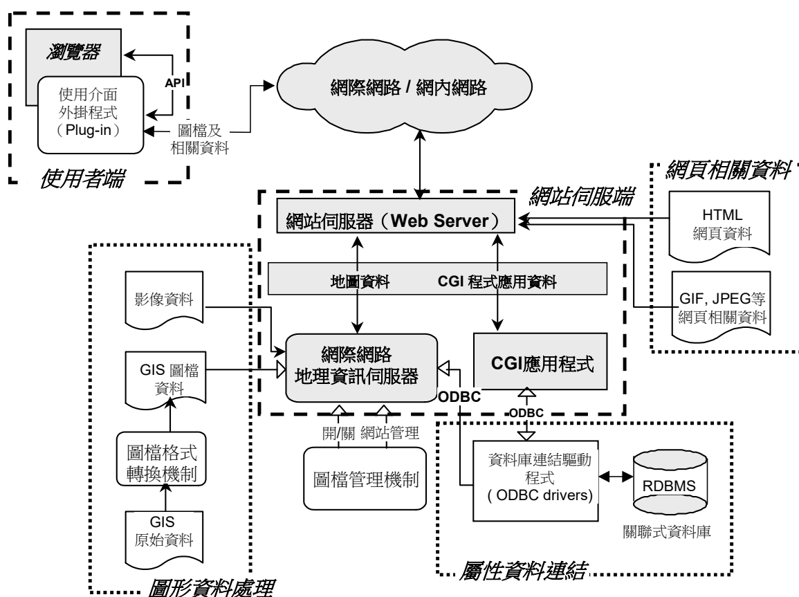
圖 3-2 網站 GIS 伺服架構圖
