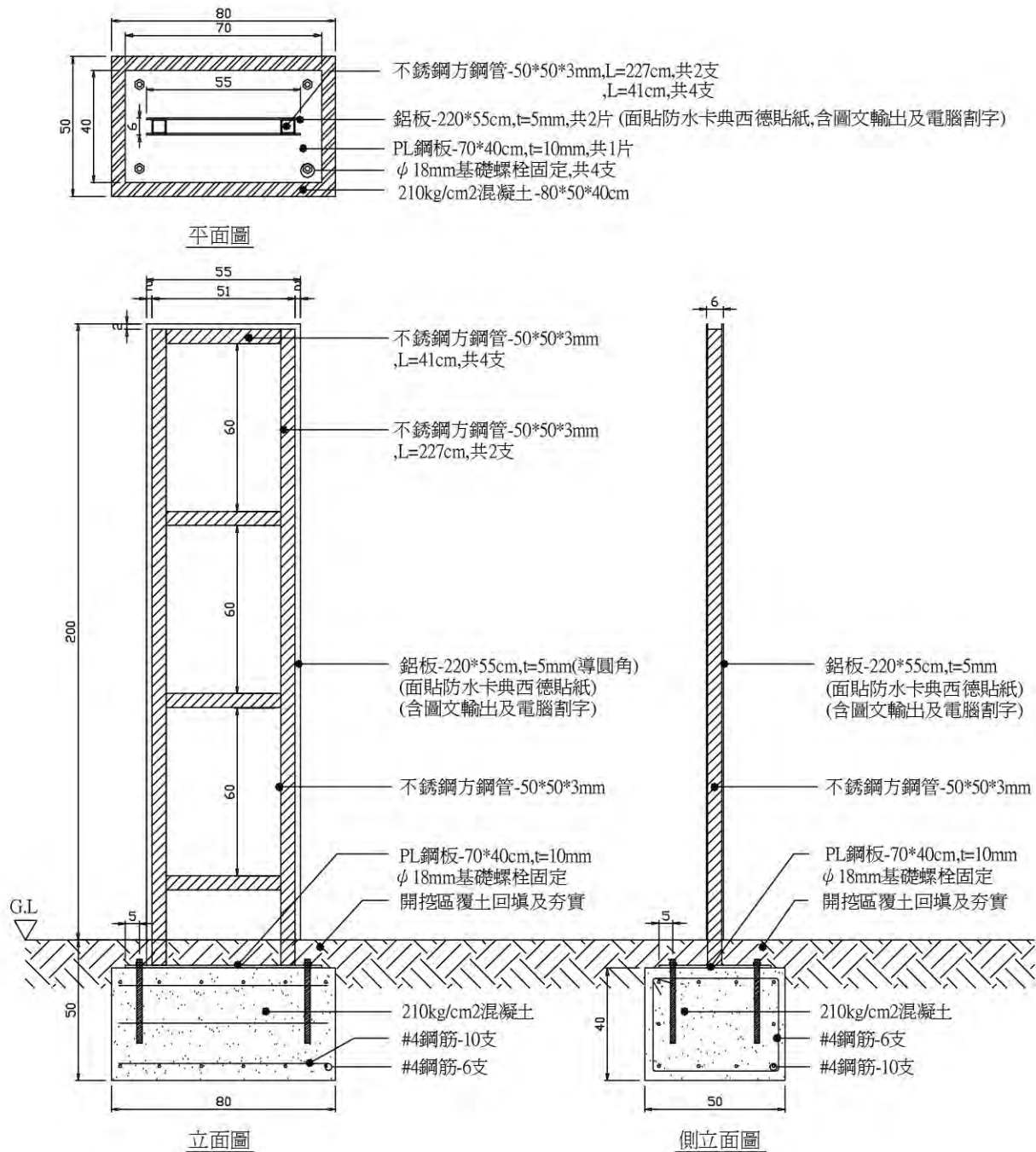
1 大型行人引導指標詳圖 E-05 說明: 鋁板與鋼管接合部使用ARGON焊接 A1:S=1/10 ; A3:S=1/20
