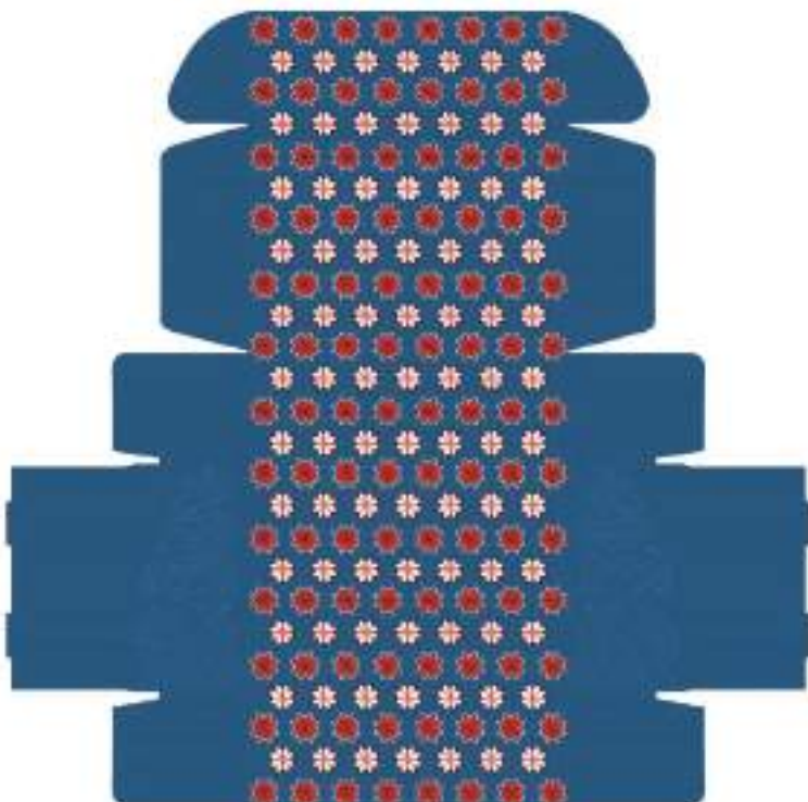
展開設計圖
