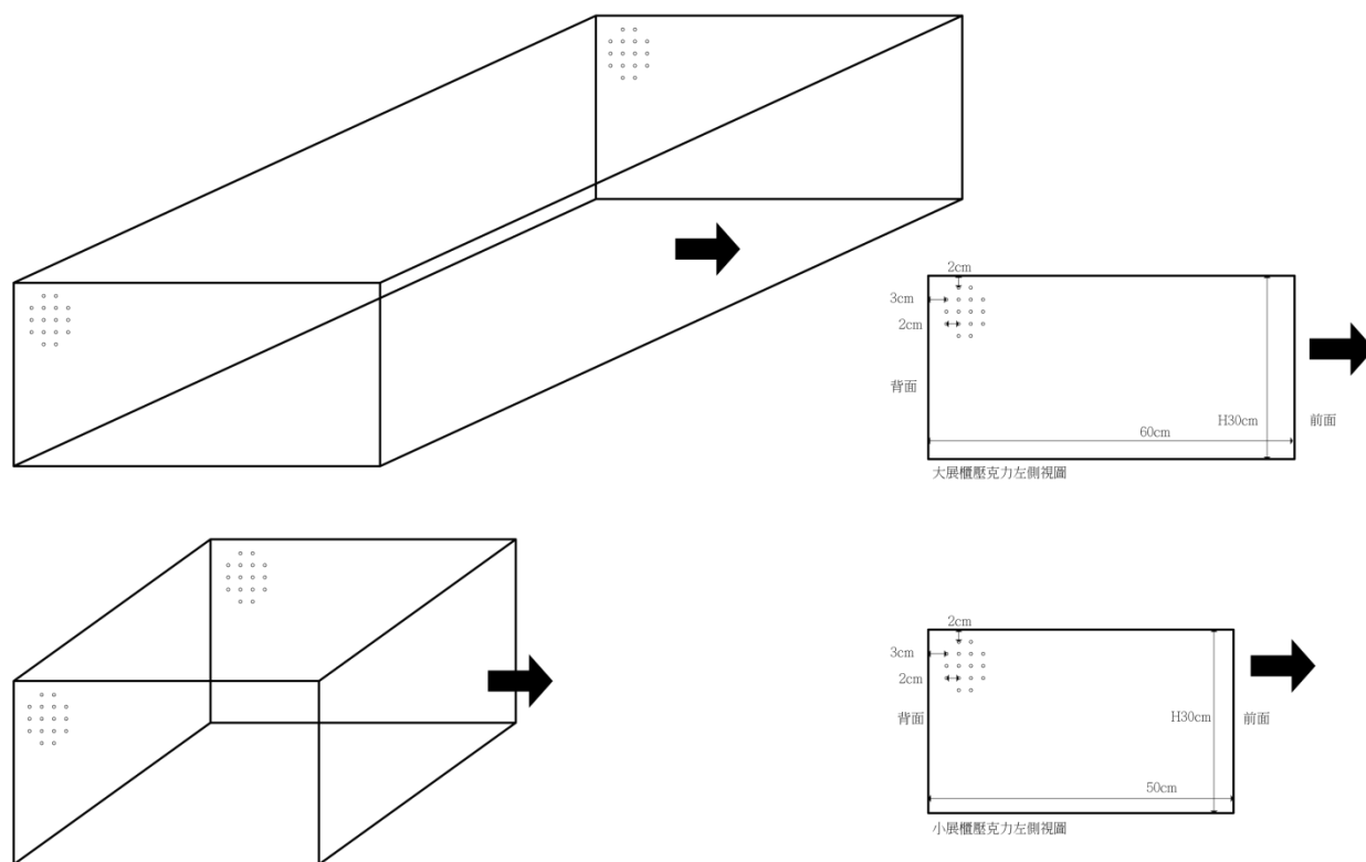
圖 2-2-1_壓克力風動圖
